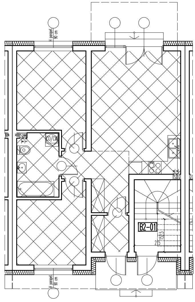
RZUT PARTERU
