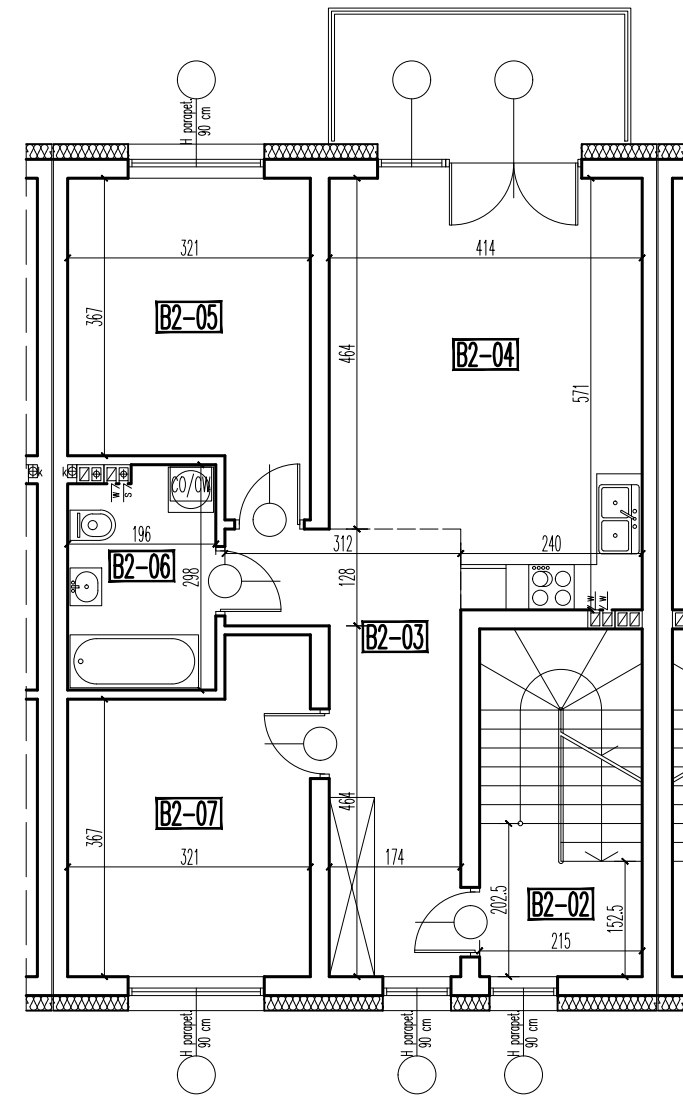
RZUT PIĘTRA
