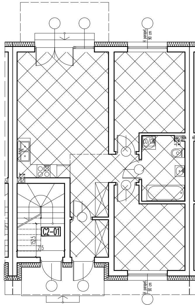
RZUT PARTERU
