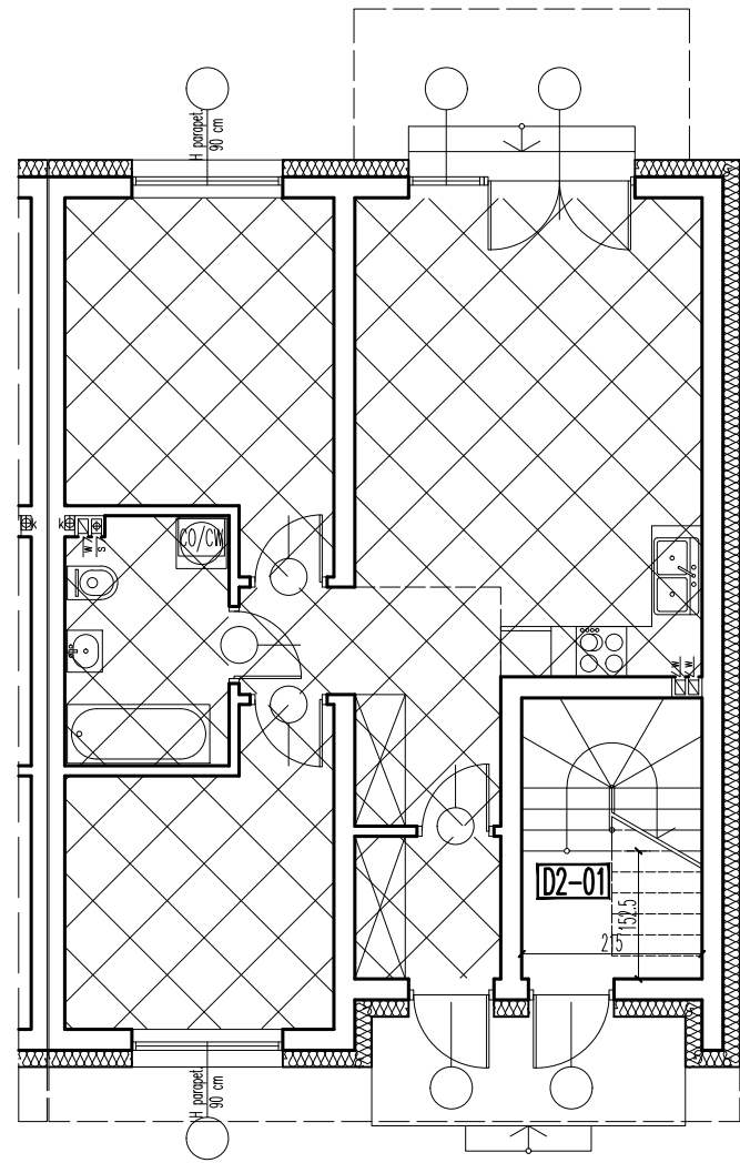
RZUT PARTERU
